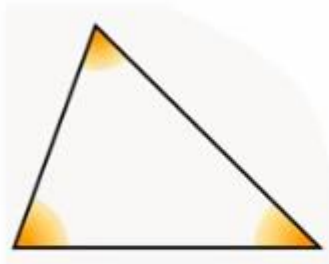
De scherphoekige driehoek
